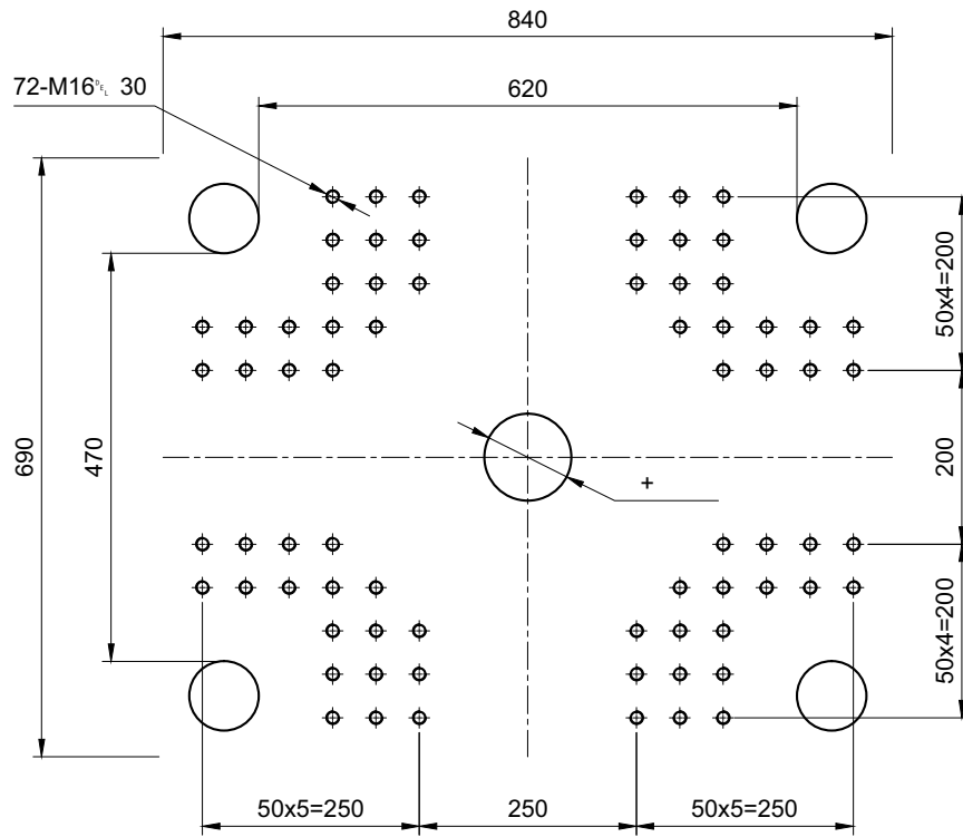
上模板 / Top Platen
