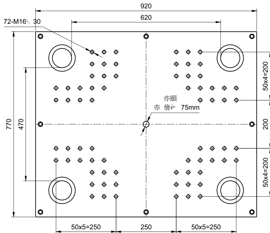
下模板 / Bottom Platen
