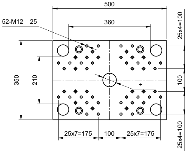
上模板 / Top Platen
