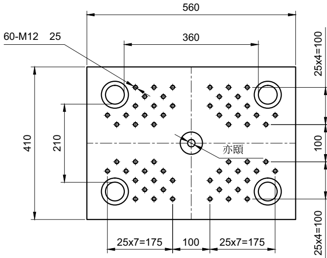
下模板 / Bottom Platen
