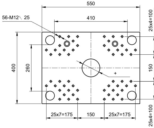
上模板 / Top Platen
