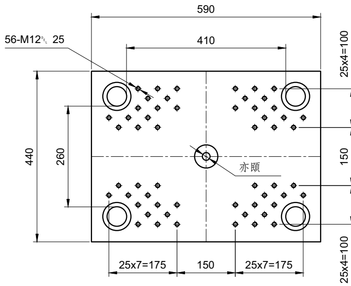
下模板 / Bottom Platen
